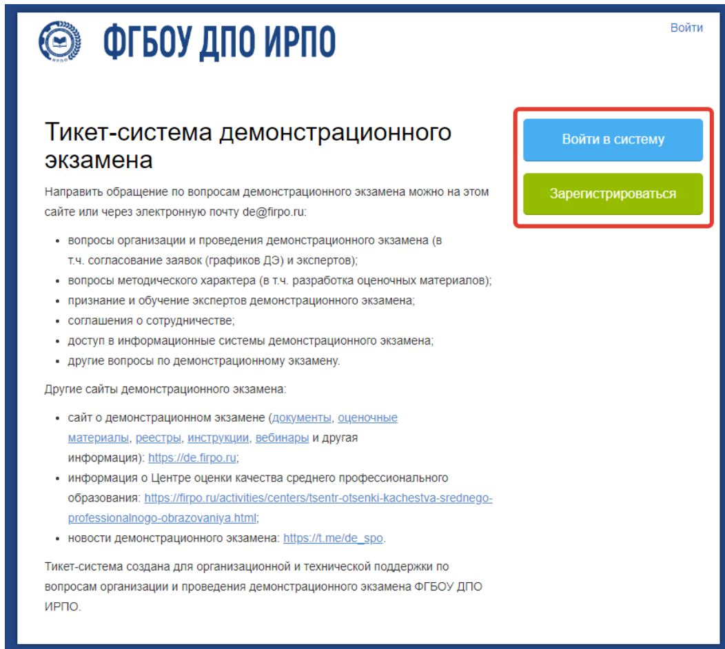
Рисунок 2 – Главная страница
